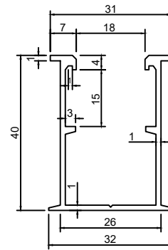
Rail nhôm Tỷ lệ: 1/1
