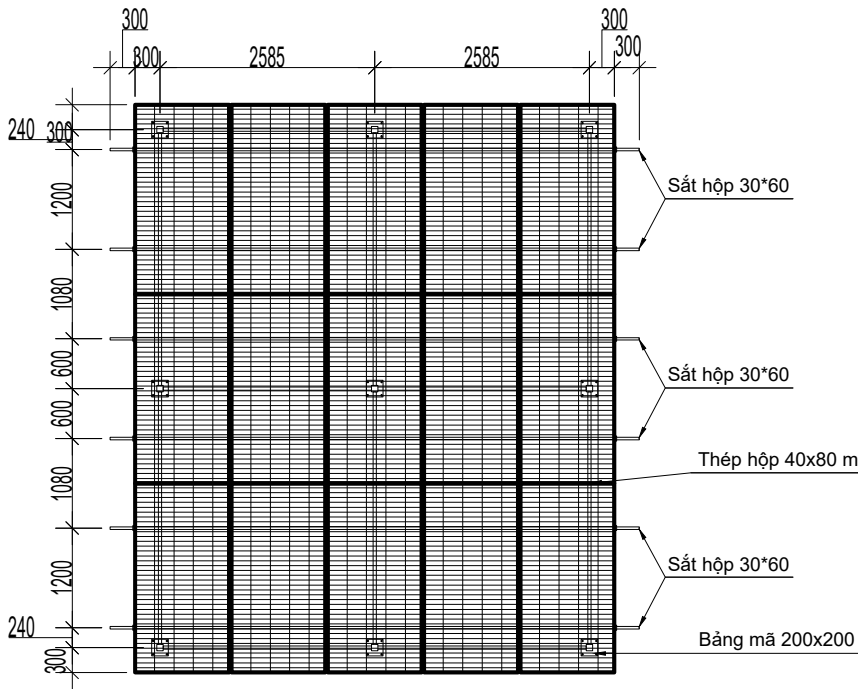
MẶT BÊN BỐ TRÍ KHUNG GIÀN TẮM PIN
