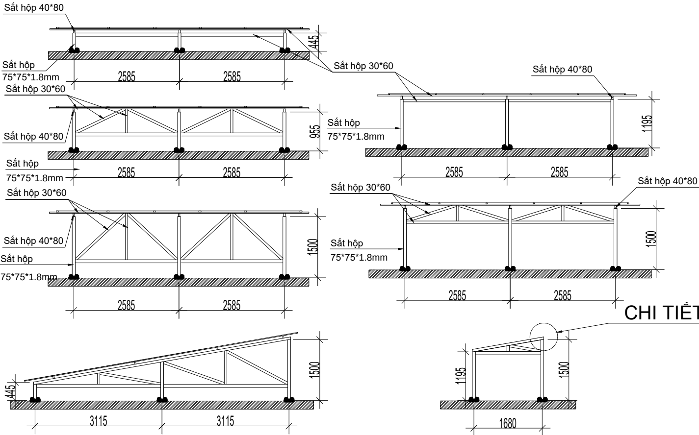
MẶT BÊN BỐ TRÍ KHUNG GIÀN TẮM PIN
