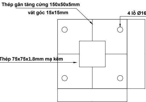
CHI TIẾT CHÂN CỘT
