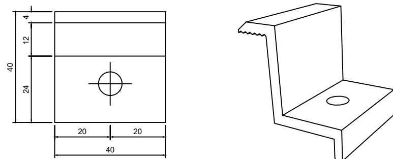
Kẹp biên Tỷ lệ: 1/1
