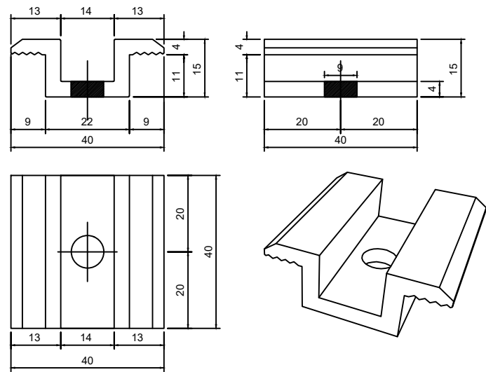
Kẹp giữa OMEGA Tỷ lệ: 1/1
