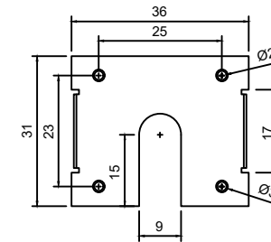
Lá tiếp địa Tỷ lệ: 1/1
