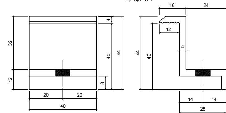
Kẹp giữa OMEGA Tỷ lệ: 1/1
