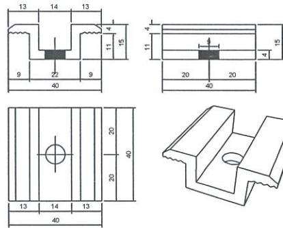
Kẹp giữa OMEGA Tỷ lệ: 1/1
