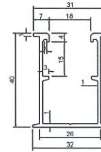
Rail nhôm Tỷ lệ: 1/1
