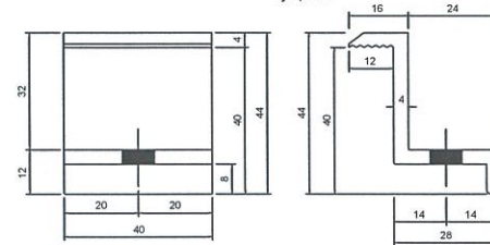
Kẹp giữa OMEGA Tỷ lệ: 1/1
