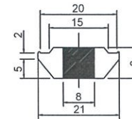
Rail nhôm Tỷ lệ: 1/1
